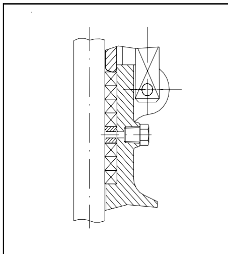
Var. 1025 Lantern ring
