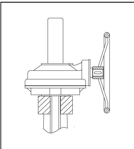
Var. 1510 Bevel gear box
